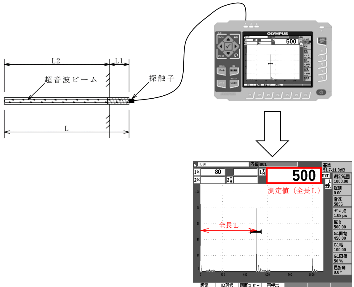
アンカーボルト長さ測定の方法
