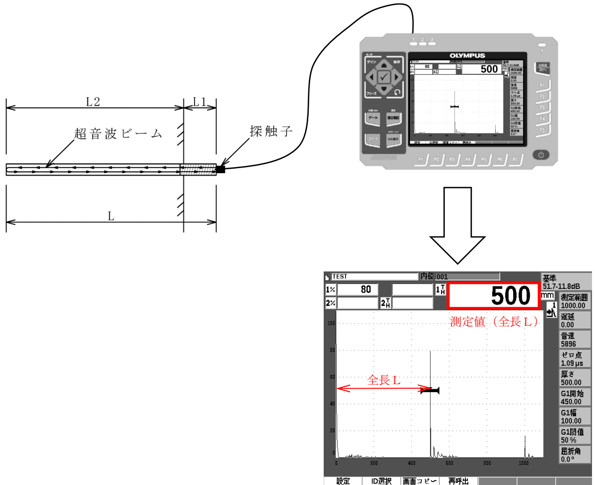
アンカーボルト長さ測定の原理
