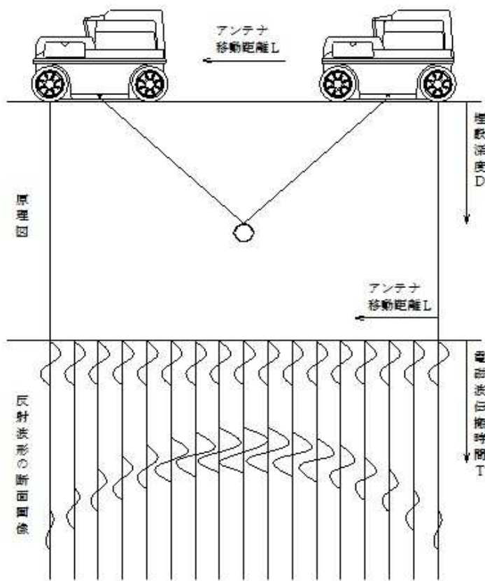
電磁波レーダー法の原理
