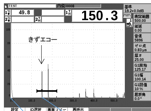
きずエコーを検出した場合の波形
