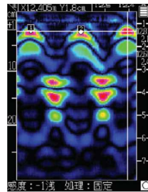
探査結果表示
