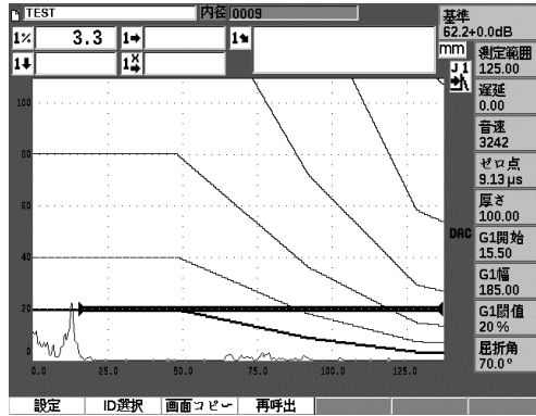
健全部の波形
