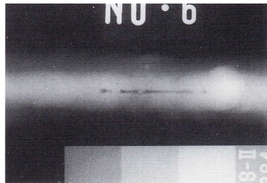
溶込み不良
